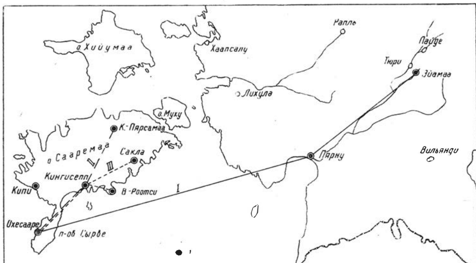
Рис. 1. Расположение приведенных на корреляционных схемах буровых скважин. Линия I — см. рис. 2; линия II — см. рис. 3; линия III — см. рис. 4. I — буровая скважина.
