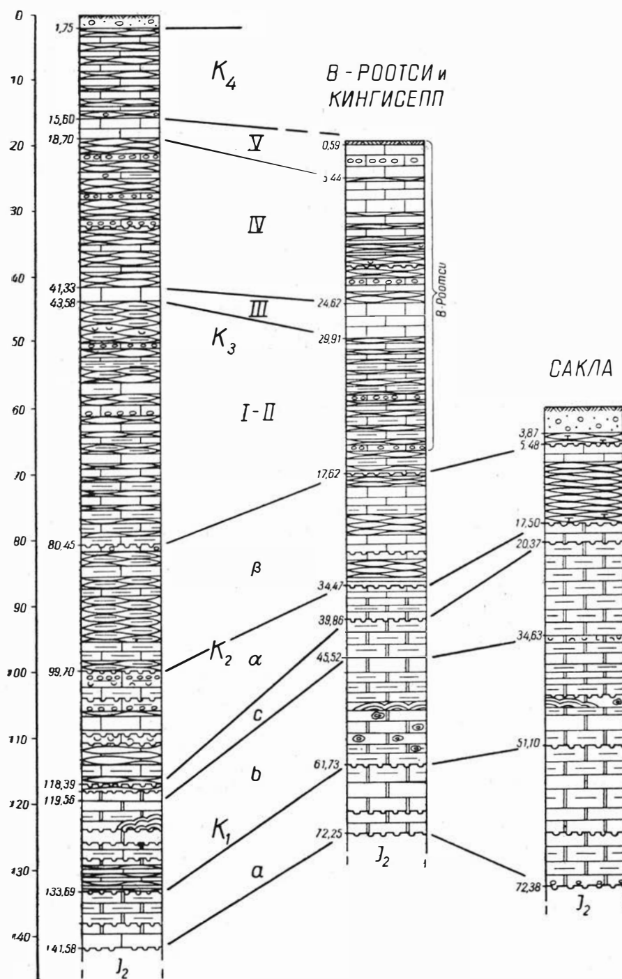
Рис. 4. Сопоставление лудловской части разрезов буровых скважин Охесааре, Вяйке-Роотси (верхняя часть средней колонки), Кингисепп и Сакла. Условные обозначения на рис. 3.
