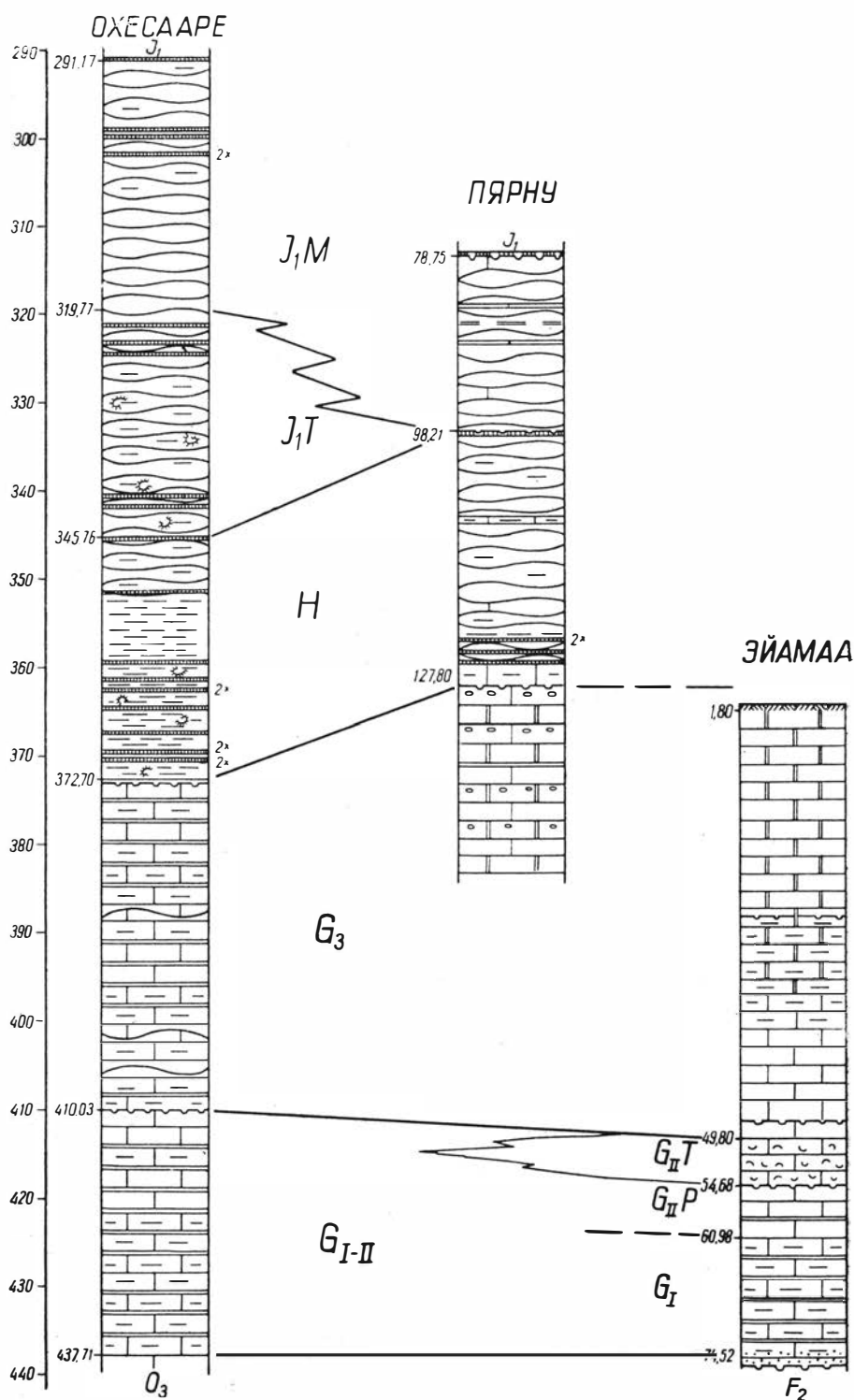
Рис. 2. Сопоставление лландоверской части и низов яниского горизонта разрезов буровых скважин Охесааре, Пярну и Эйамаа. Условные обозначения на рис. 3.
