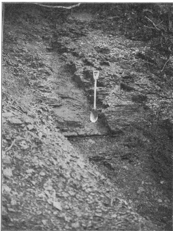
Fig. 2. Öfre och mellersta delen af lokal E 15 , Fågelsång.
