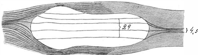
Fig. 14. Orstenboll i skiffern vid lokal 3 å Andersön. Skala 1:3.
