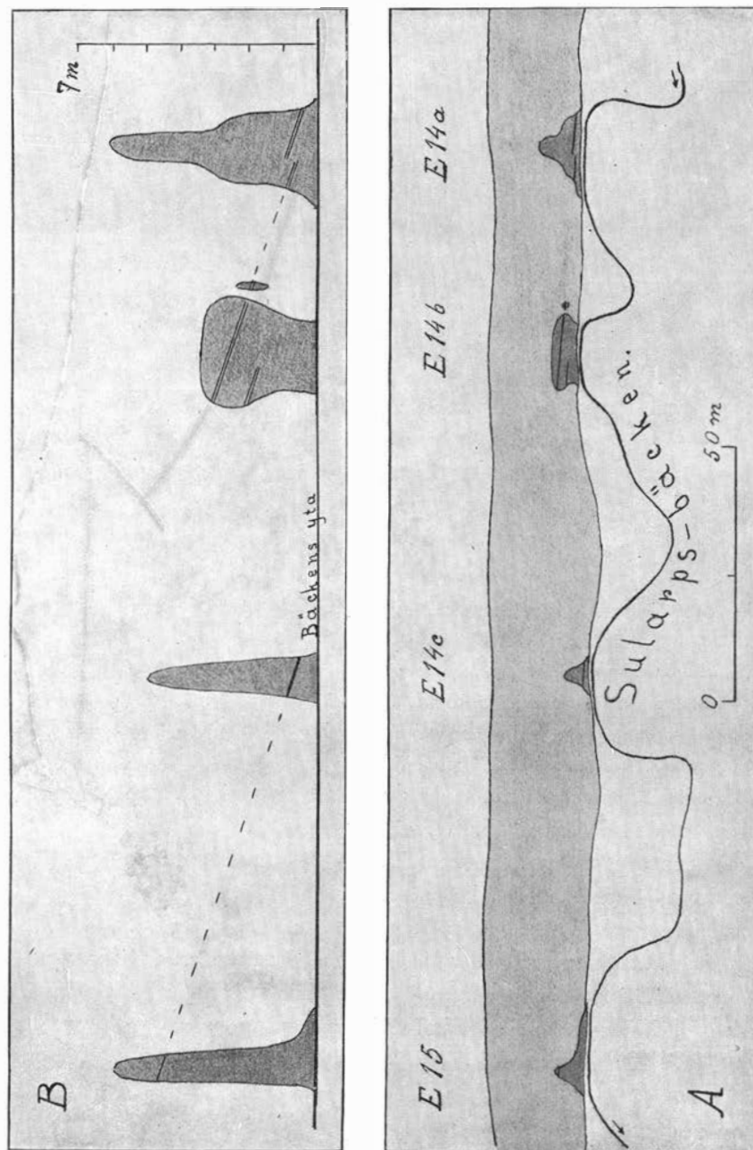
Fig. 3. A. Kombinerad plan- och perspektivskiss öfver lokalerna E 15 och E 14 a—c. Höjd- och längdskala lika. B. Profilleckning af samma lokaler. Höjdskalet omkring 7 ggr längdskalan.
