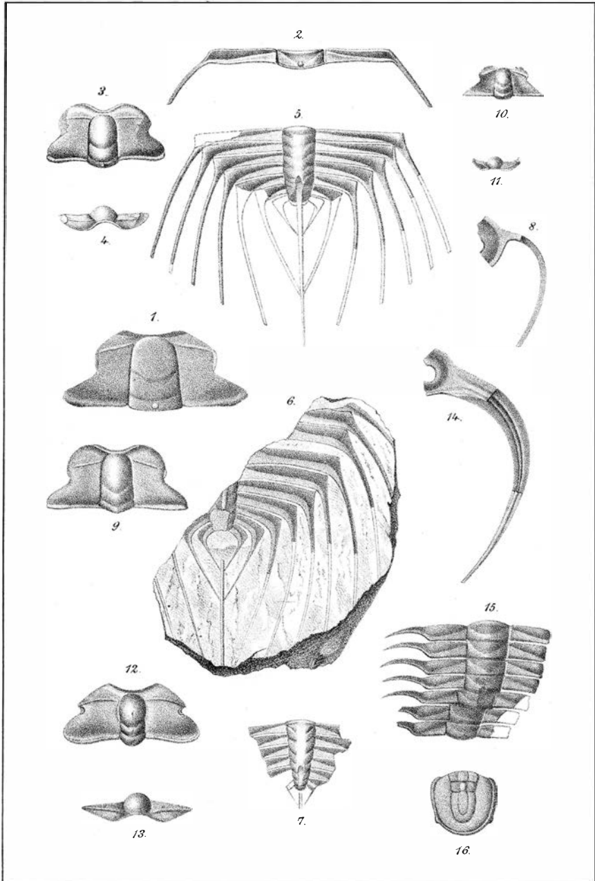
1, 2. Ctenopyge bisulcata . 3-9. Ctenopyge pecten . 10, 11. Ctenopyge concava . 12, 13. Ctenopyge teretifrons 14, 15. Ctenopyge sp. indet. ? 16. Agnostus trisectus .
