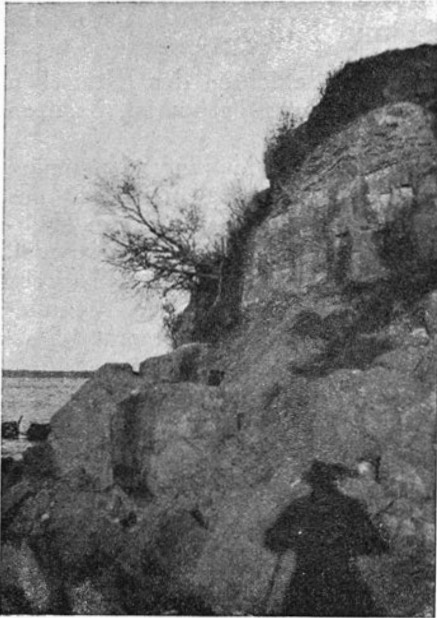
Fig. 2. Marienberg bei Tallinn (Reval). Sandsteine der Scenella -Zone mit quadri-ger Absonderungsform. Allgemeine Ansicht: Oben — die Schichten der Scenella -Zone, niedriger — die tonigen Schichten der unteren Zone. Am Strande liegen die Sandsteinquadern, welche aus der oberen ( Scenella )-Zone stammen.
