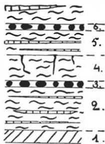
Fig. 5. Marienberg. Profil der unteren Zone des Eophyton -Sandsteines, entspricht der Abb. 3. 1. Glaukonitreicher Sandstein und Ton mit Mesonacis -Bruchstücken, liegt am Meeresspiegel. 0,1—0,15 m. 2. Abwechselnd Ton- und Sandsteinschichten mit zahlreichen Volborthella tenuis . — 1,0 m. 3. Konglomerat mit Volborthella 0,08 m. 4. Ton mit Trockenrissen, die eine Tiefe von 0,4 m erreichen und stellenweise mit Volborthellen gefüllt sind (Abb. 1, Taf. II). 0,5 m. 5. Dünnschichtige Sandsteine und Tone mit Volborthella tenuis 0,4—0,6 m. 6. Konglomerat mit grossem Geröll und zahlreichen Volborthellen . 0,1 m. Höher — Sandsteine und Tone mit Cruciana , Fraena usw. Schutt.
