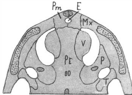
Fig. 6. Pareiasaurus bombidens SEELEY. Nach WATSON (11. S. 160). Gaumen von oben gesehen. \frac{1}{6} der natürl. Grösse.
