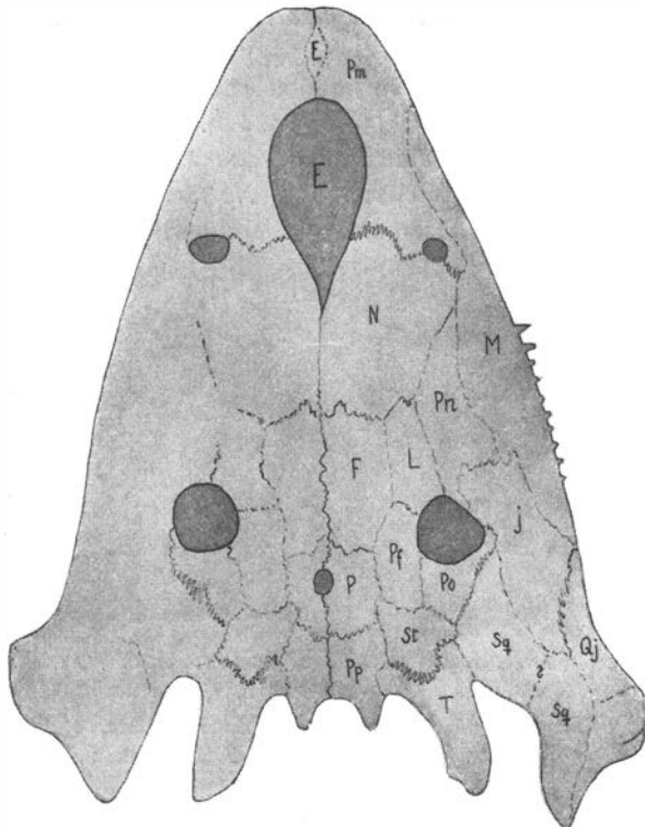
Fig. 5. Dasyceps Bucklandi LLOYD. Nach v. HUENE. \frac{1}{3} der natürl. Grösse.
