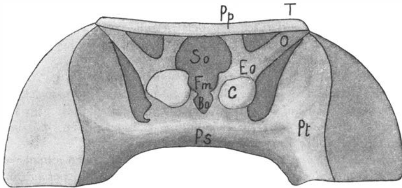
Fig. 2. Tertrema acuta . Hinterhaupt, teilweise ergänzt. \frac{1}{2} der natürl. Grösse. Pp Postparietale, T Tabulare, So Supraoccipitale und Bo Basioccipitale, Fm Foramen magnum, C Condylus, Eo Exoccipitale, O Opisthoticum, Pt Pterygoideum, Ps Parasphenoideum.
