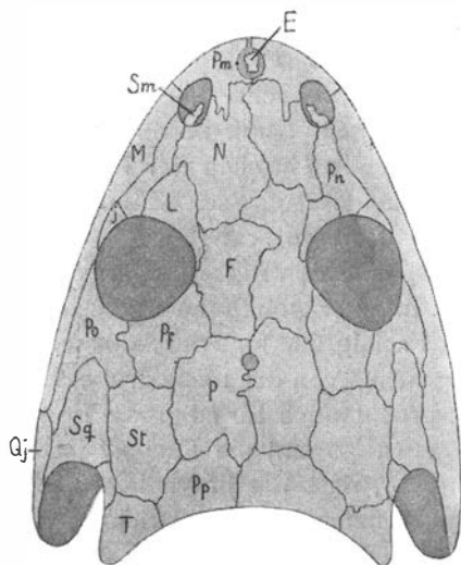
Fig. 3. Micropholis Stowi HUX. nach WATSON. Vergr. \frac{3}{2} .
