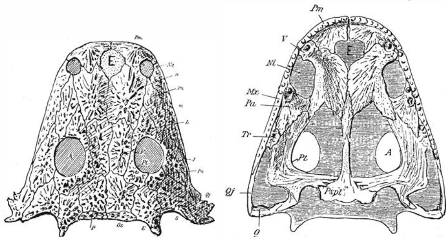
Fig. 4. Acanthostoma vorax CRED. Nach JAEKEL. (6. S. 115) \frac{2}{3} der natürl. Grösse.
