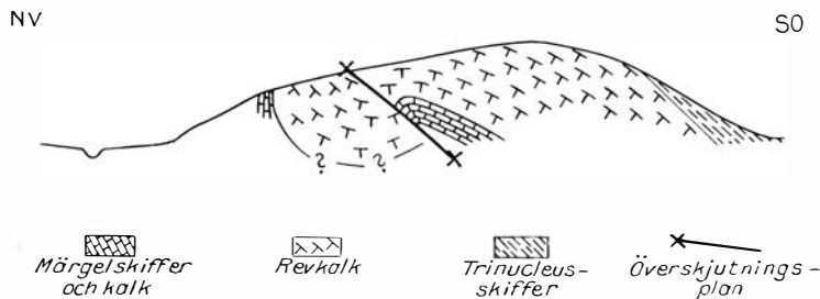
Fig. 10. Profil genom kalkstenskullen vid Sättra. Sannolik rekonstruktion av berggrundens byggnad
