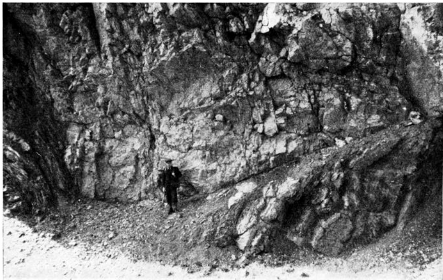
Fig. 12. Överskjutningen vid ingången till kalkstensbrottet vid Kullberg. Under och till höger om mannen, som står på överskjutningsplanet, synas de inverterade trinucleuslagren, ovanför grovbrecierad revkalk. — B. Bohlin foto.
