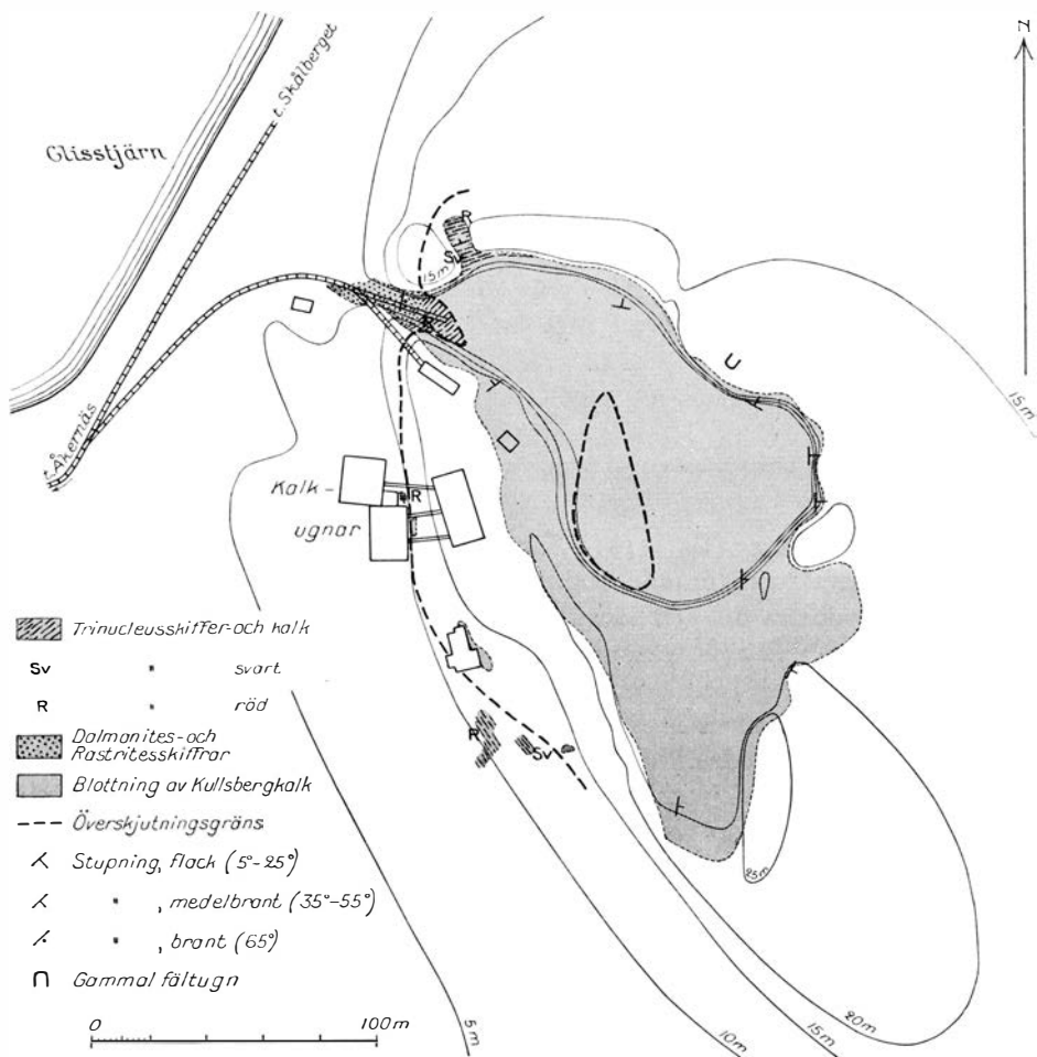
Fig. 11. Karta över Kullbergområdet.
