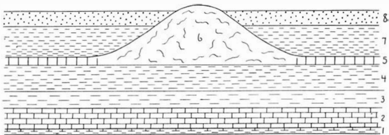
Fig. 5. Schematisk framställning av lagserien inom Siljansområdet enligt Nathorsts revteori för leptanakalken (efter Nathorst). 1 = ceratopygeled, 2 = ortocerkalk, 3 = chasmopsled, 4 = trinucleusled, 5 = klingkalk, 6 = leptanakalk, 7 = övre graptolitskiffrar, 8 = slipsandsten.
