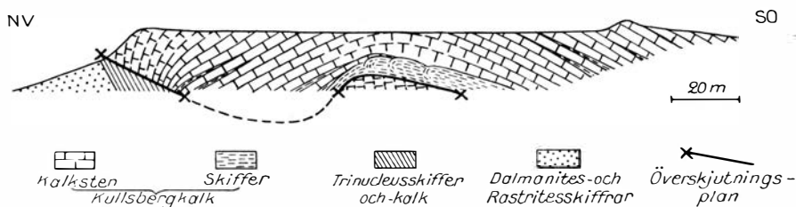
Fig. 13. Något schematiserad profil genom Kullberget.
